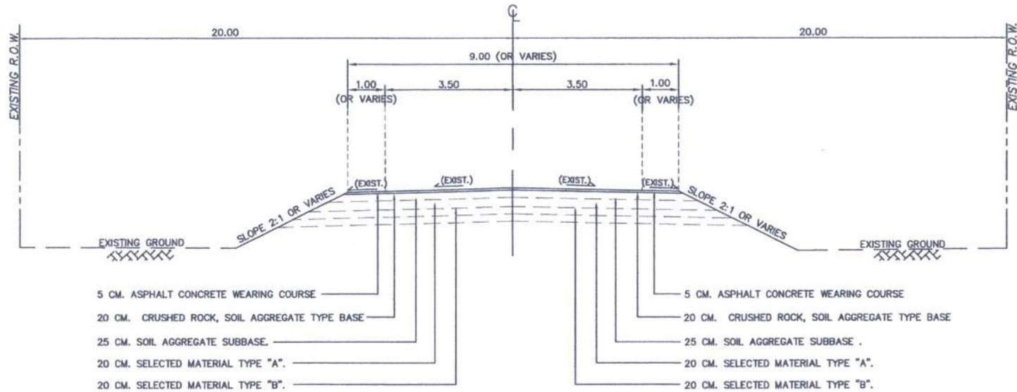
TYPICAL CROSS SECTION (ก่อนทำการปรับปรุง)
