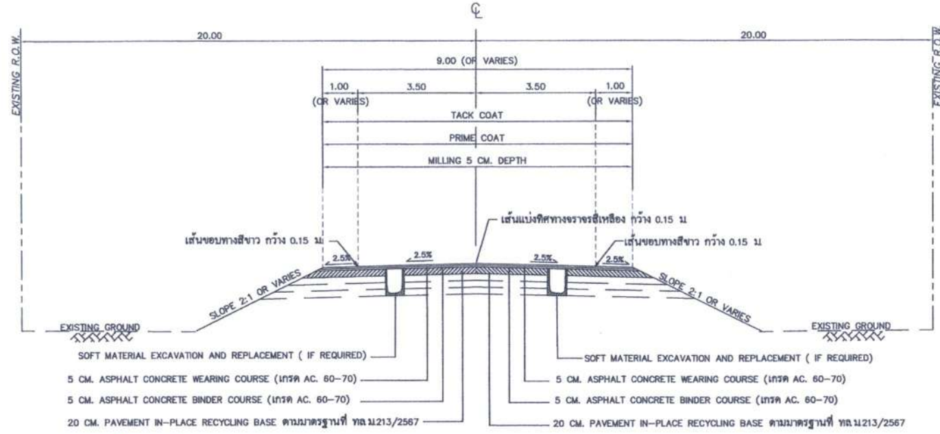
TYPICAL CROSS SECTION (หลังทำการปรับปรุง) กม.158+465.000 - กม.160+075.000 NOT TO SCALE
