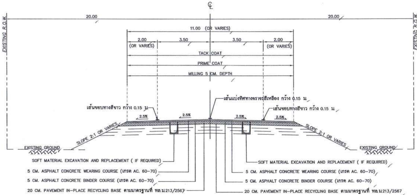
TYPICAL CROSS SECTION (หลังทำการปรับปรุง) กม.50+760.000 - กม.52+014.000 NOT TO SCALE
