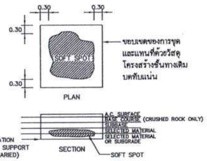
รูปแสดงการแก้ไขบริเวณจุดอ่อนตัว (SOFT SPOT)
