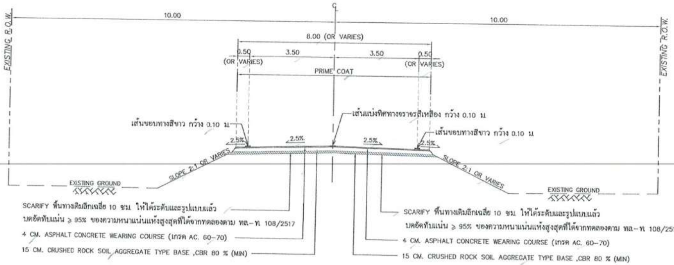
TYPICAL CROSS SECTION (หลังทำการปรับปรุง) กม. 84+085.000 - กม. 87+000.000 NOT TO SCALE
