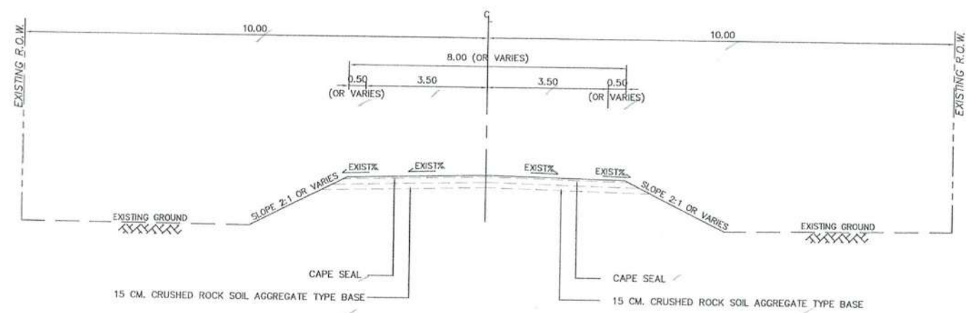
TYPICAL CROSS SECTION (ก่อนทำการปรับปรุง) กม. 84+085.000 - กม. 87+000.000 NOT TO SCALE
