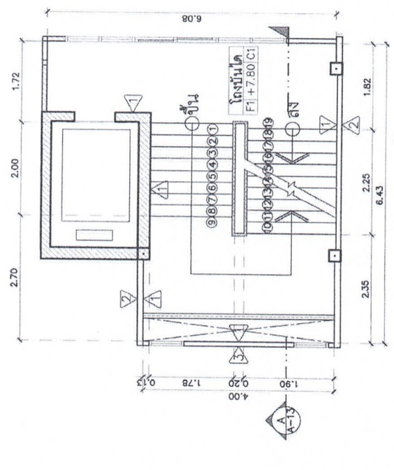
แบบตัดหน้า 3 SCALE 1:75
