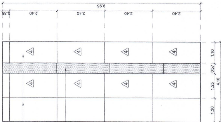
รูปด้าน 2 SCALE 1:75
