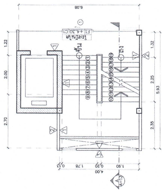
แบบตัดหน้า 2 SCALE 1:75
