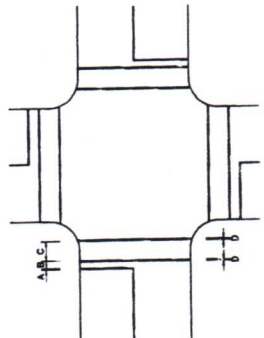
A = 0.30-0.60 M. B = 1.00 M. C = 2.00-4.00 M. D = 0.5 A. E = 0.80 M. F = 0.60 M.
