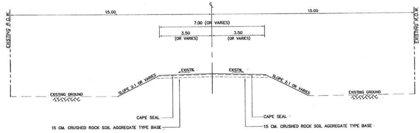
TYPICAL CROSS SECTION (ก่อนการปรับปรุง) กม.31+000.000 - กม.34+165.000 NOT TO SCALE
