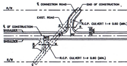
RIGHT OF WAY WIDTH > 20.00\text{M} (NOT EXCEED 30.00 M.) : R=8.00 M. R'=8.00 M. RIGHT OF WAY WIDTH > 30.00 M. : R=5.00M(MIN.) R'=15.00 M(MIN.)
