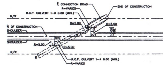
RIGHT OF WAY WIDTH \leq 20.00 M.
