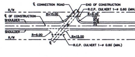
RIGHT OF WAY WIDTH \leq 20.00 M.
