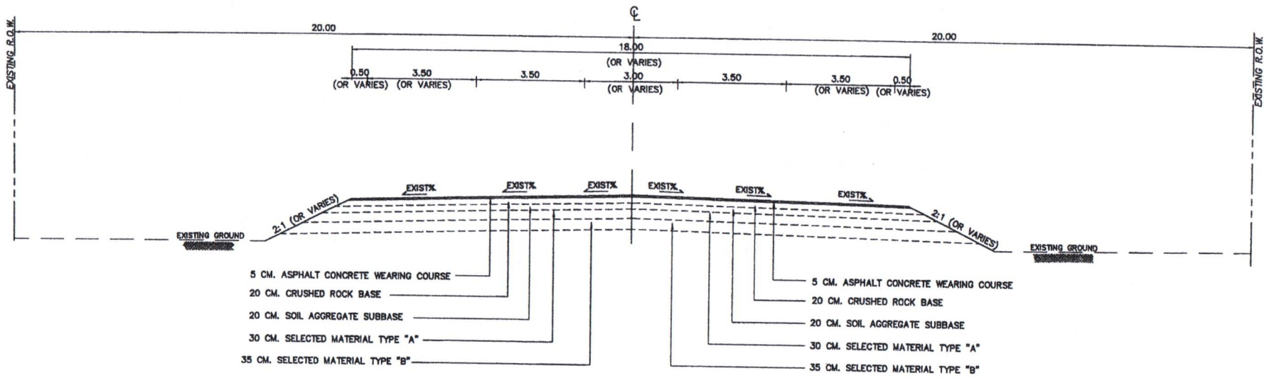
TYPICAL CROSS SECTION (ก่อนการปรับปรุง) กม.0+000.000 - กม.0+155.000 NOT TO SCALE
