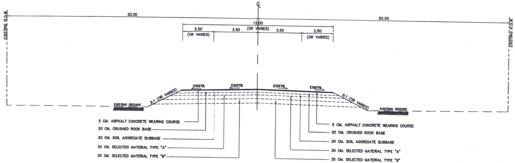
TYPICAL CROSS SECTION (ก่อนการปรับปรุง) กม.0+155.000 ~ กม.2+755.000 / NOT TO SCALE
