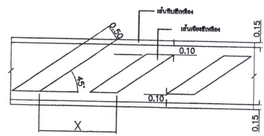
รูปขยายเส้นแบ่งทิศทางจราจร NOT TO SCALE
