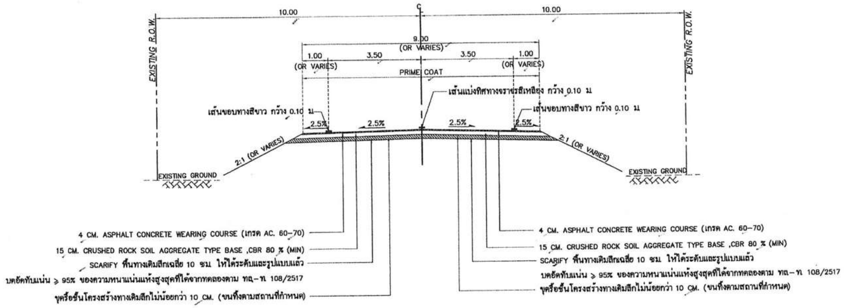
TYPICAL CROSS SECTION (หลังการปรับปรุง)
