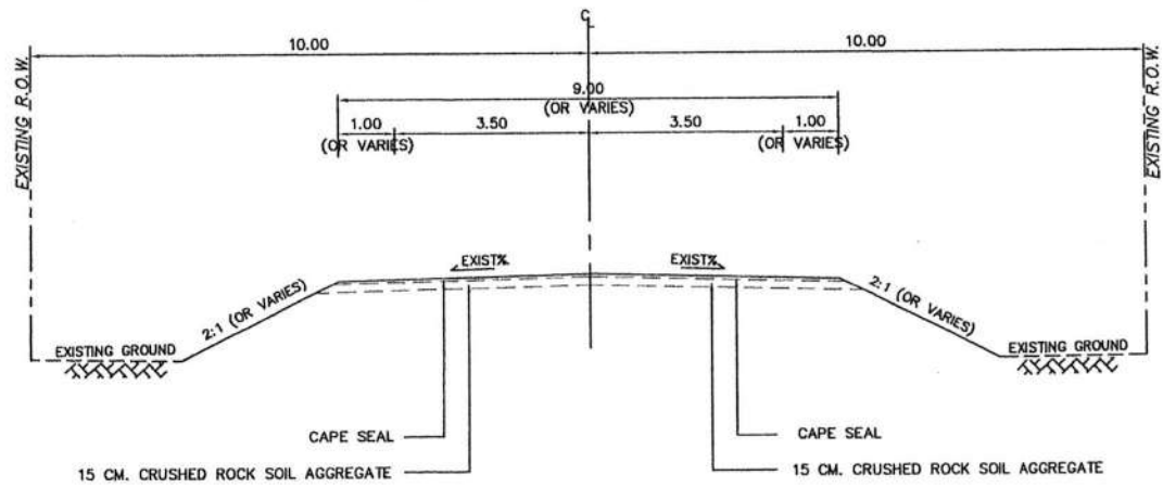
TYPICAL CROSS SECTION (ก่อนการปรับปรุง)
