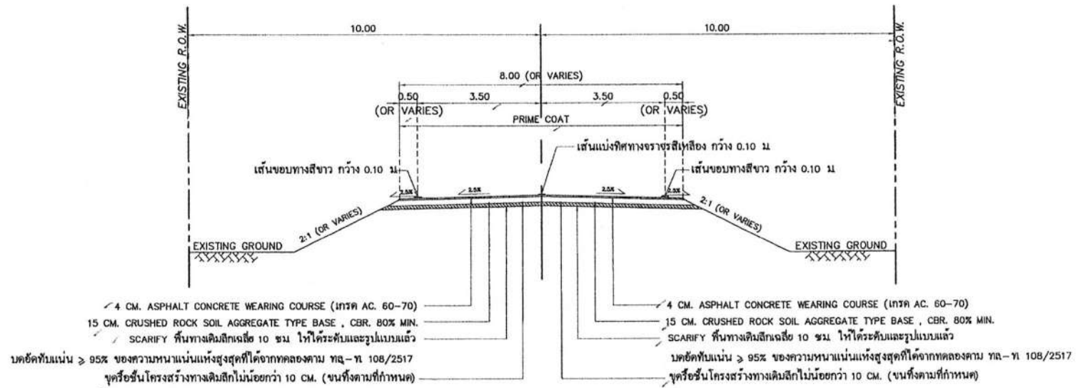
TYPICAL CROSS SECTION (หลังการปรับปรุง) กม.11+551.000 - กม.14+450.000 NOT TO SCALE
