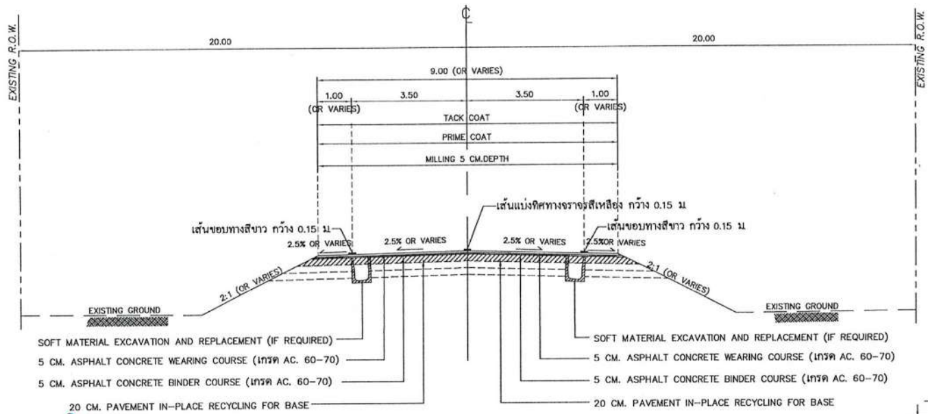
TYPICAL CROSS SECTION (หลังทำการปรับปรุง) กม.168+500.000 - กม.170+122.000 NOT TO SCALE
