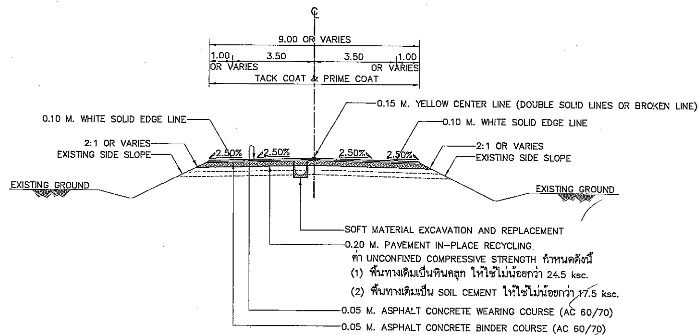
TYPICAL CROSS SECTION (หลังปรับปรุง)
