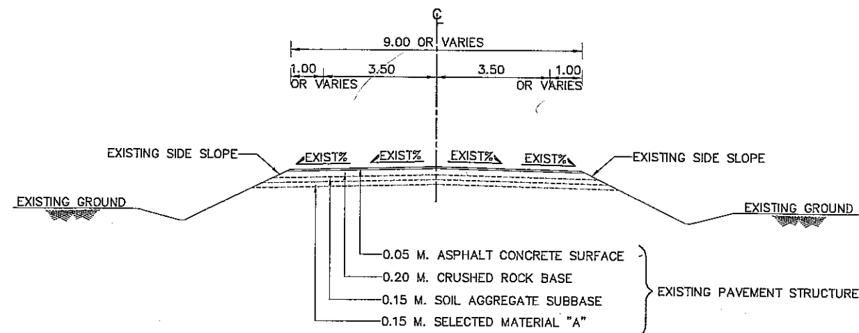
TYPICAL CROSS SECTION (ก่อนปรับปรุง)
