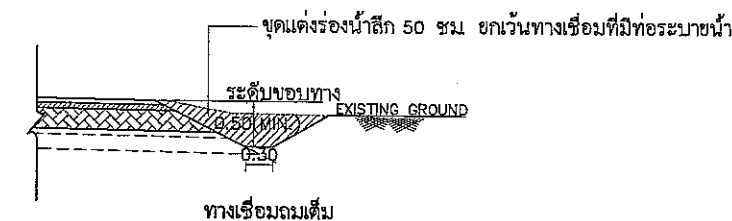
แบบขยายการปรับปรุงระบบระบายน้ำข้างทาง
