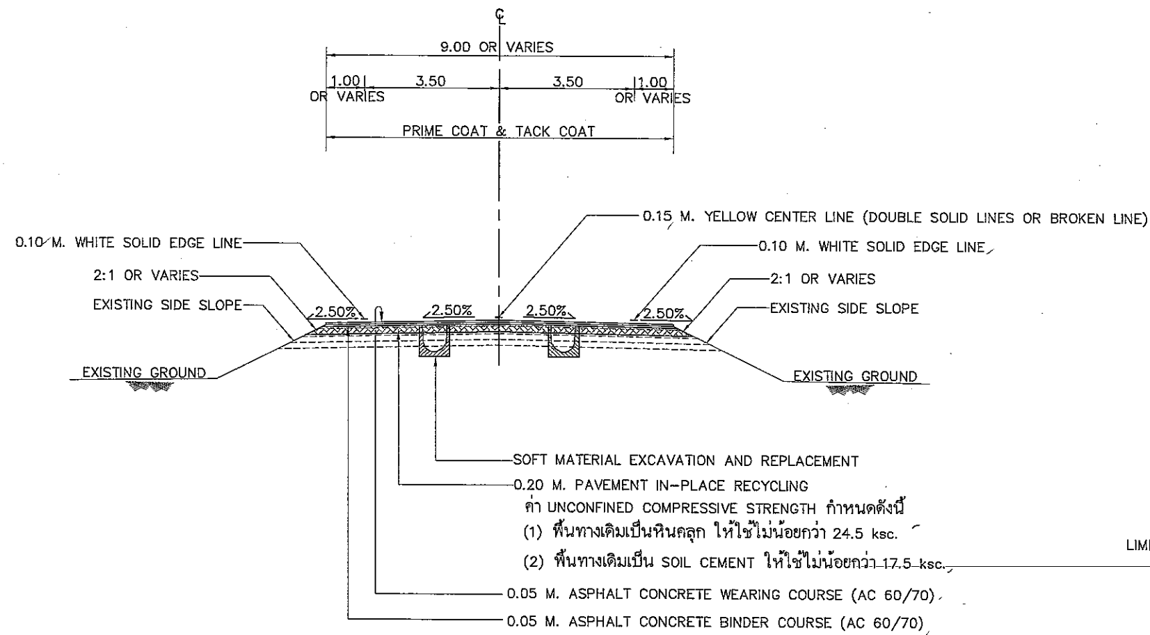
TYPICAL CROSS SECTION (หลังปรับปรุง)
