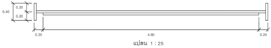
รูปด้านหน้า 1 : 25
