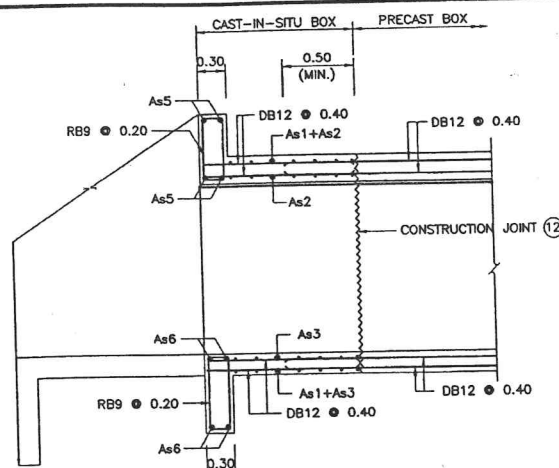
SECTION A - A SCALE 1 : 100
