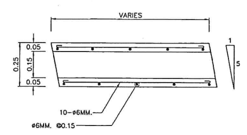
SECTION (D) - (D) SCALE 1 : 10
