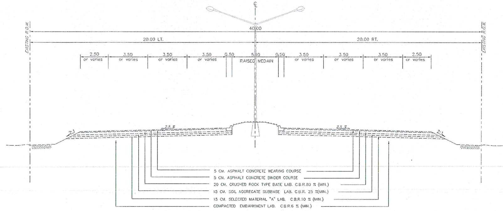
TYPICAL CROSS - SECTION ระหว่าง กม.974+727 - กม.974+905 (LT.) (ก่อนปรับปรุง)
