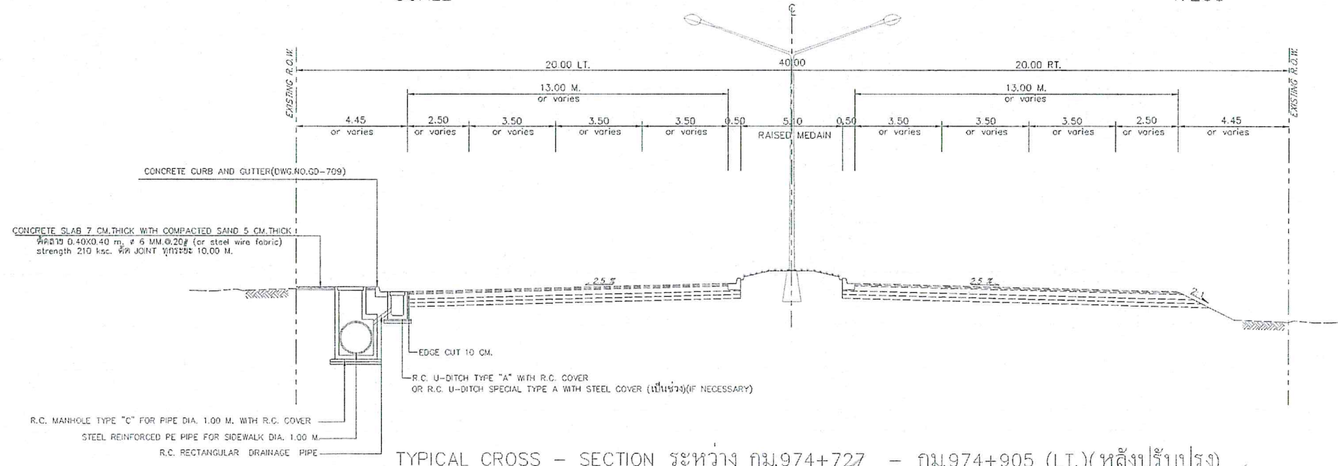
TYPICAL CROSS - SECTION ระหว่าง กม.974+727 - กม.974+905 (LT.) (ก่อนปรับปรุง)
