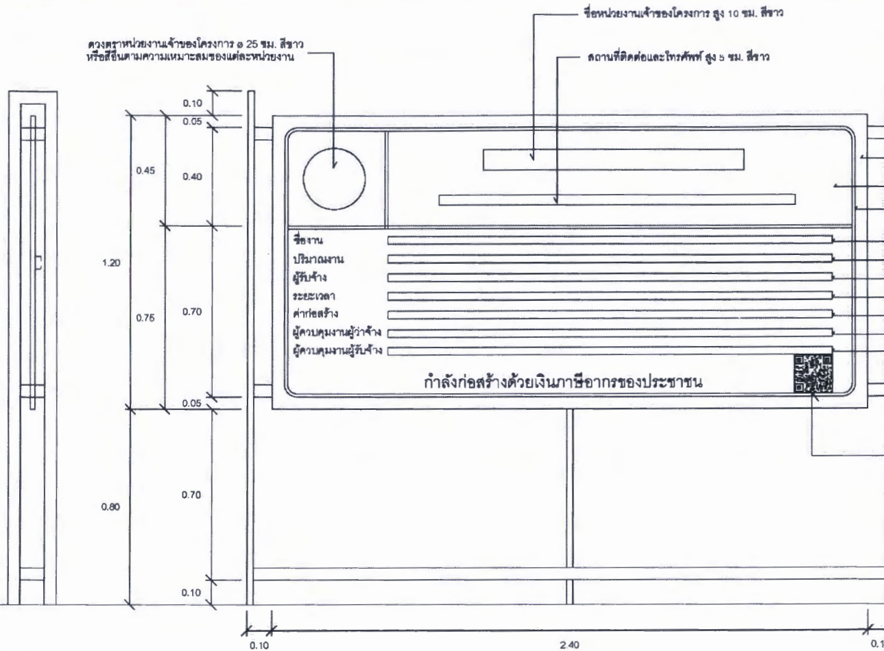
รูปด้านข้าง 1 : 50
