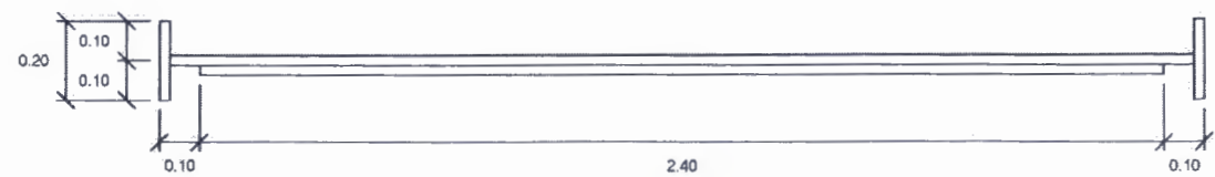
แปลน 1 : 50
