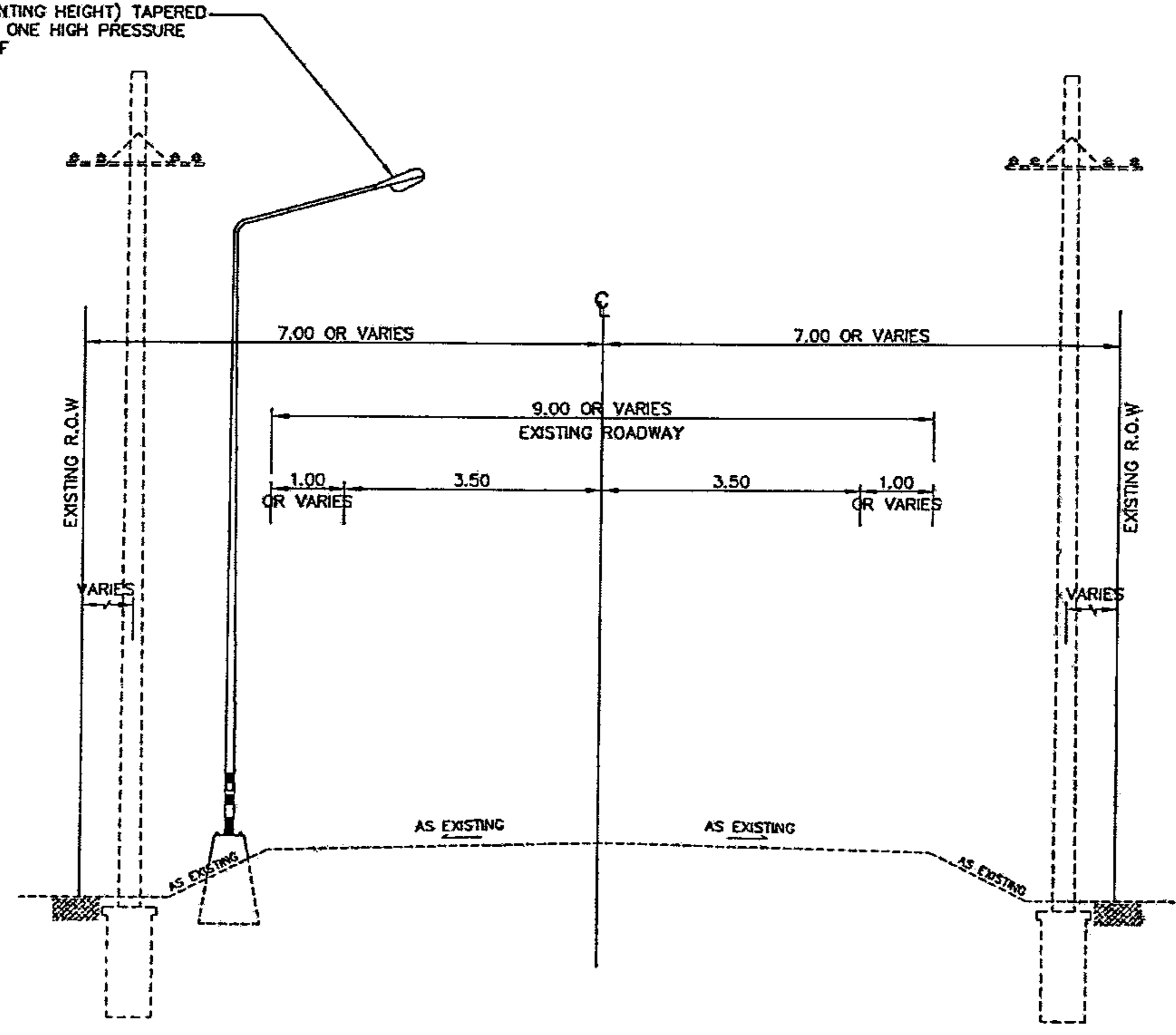
TYPICAL CROSS SECTION I SCALE 1:100 กม+500 - กม+698 (เป็นช่วงๆ)
