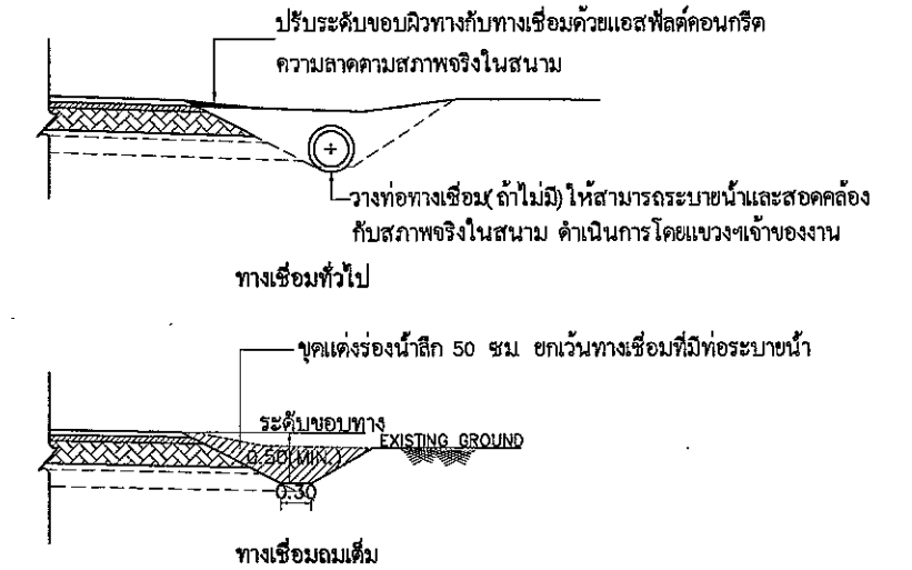
แบบขยายการปรับปรุงระบบระบายน้ำข้างทาง
