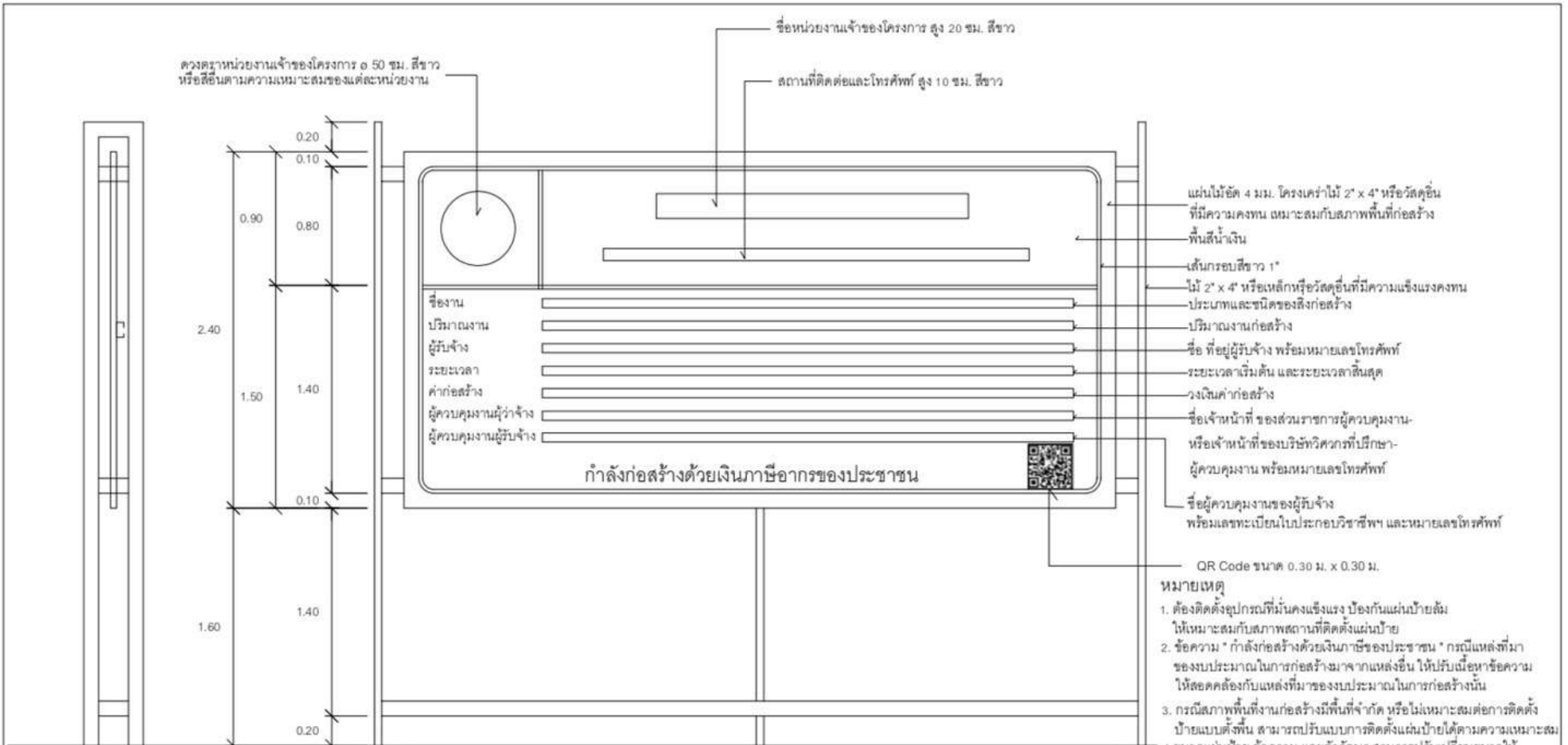
รูปด้านหน้า 1 : 25
