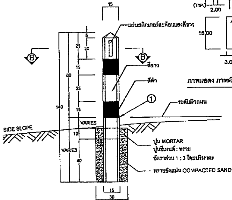
ภาพแสดง เสาเหล็กนำทางยางพารา (ด้านหน้า)
