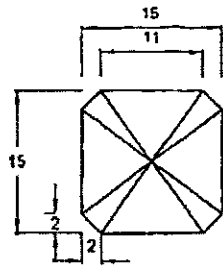
ภาพแสดง มุมมองจากด้านบนอุปกรณ์เสาลักน้ำทางยางพารา
