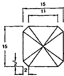
ภาพแสดง เสาเหล็กนำทางยางพารา (ด้านบน)
