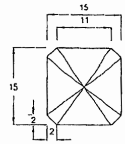
ภาพแสดง เส้นลึกลงทางยางพารา (ด้านบน)
