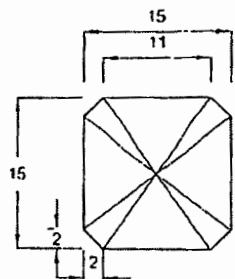
ภาพแสดง มุมมองจากด้านบนอุปกรณ์เสาหลักนำทางยางพารา
